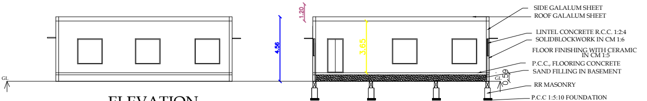
ELEVATION
