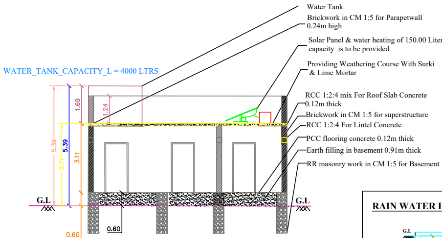
SECTION A-B
