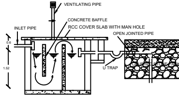
LONGITUDINAL SECTION
