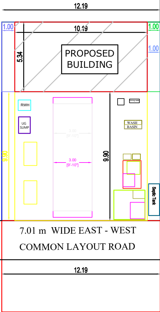
SITE PLAN (Scale : 1:100)
