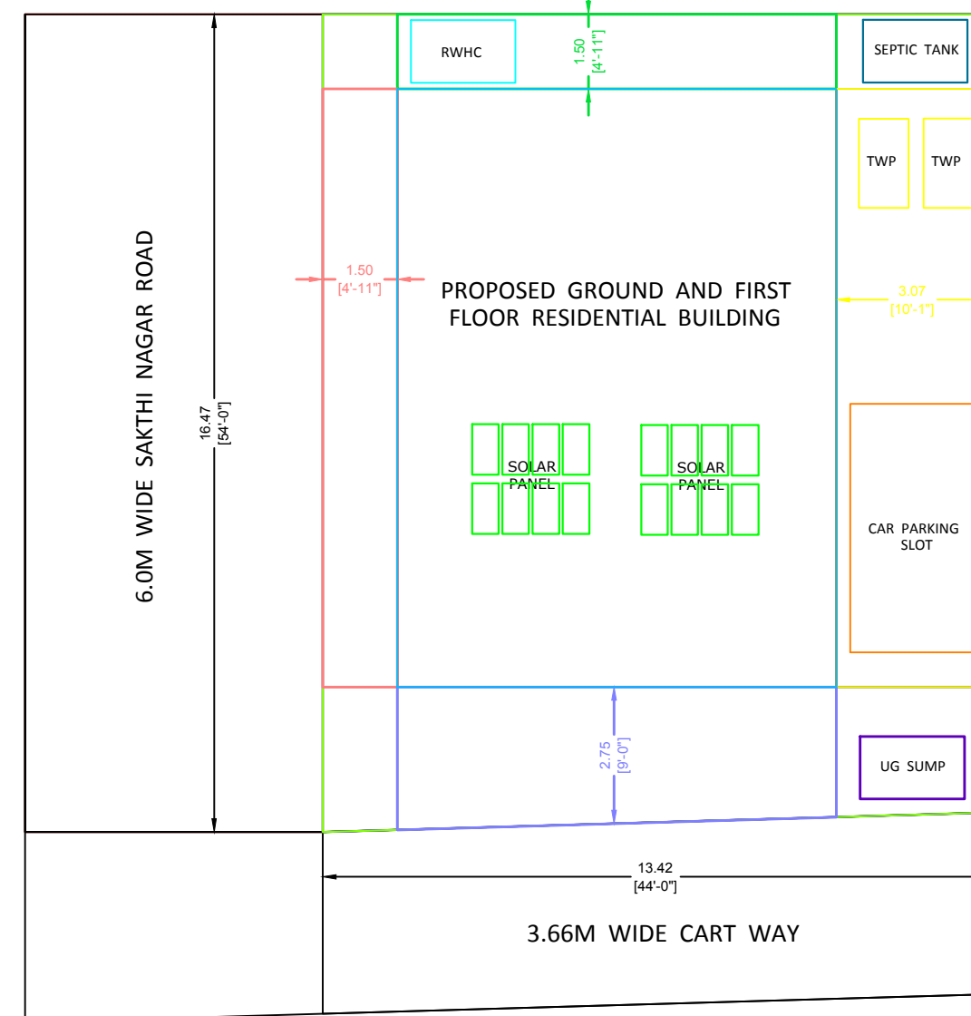
SITE PLAN 1 : 100
