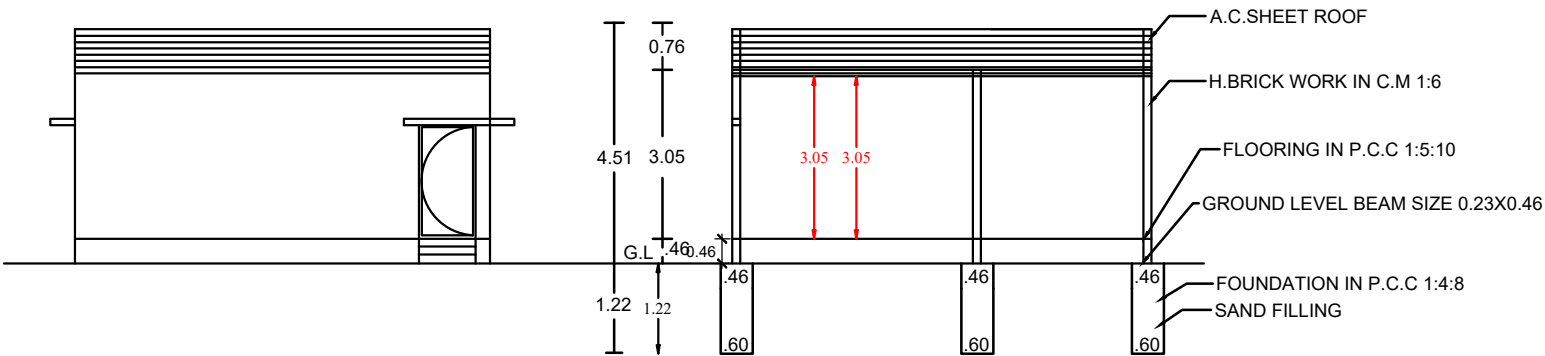
ELEVATION
