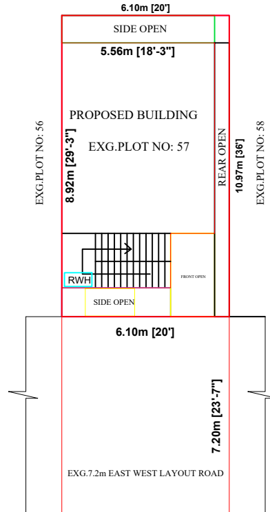
SITE PLAN SCALE : 1:100
