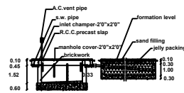
LONGITUDINAL SECTION
