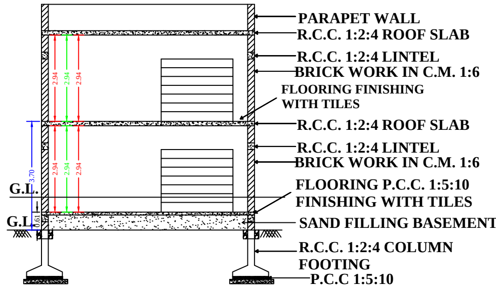
SECTION A-A
