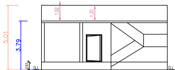
ELEVATION
