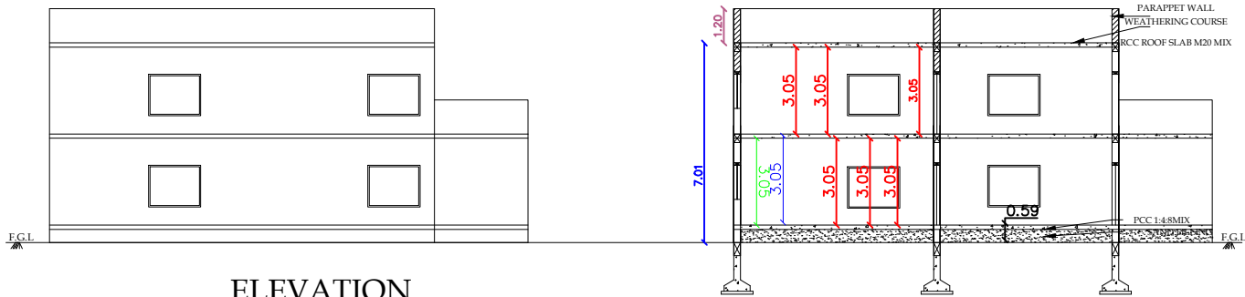
SECTION A-A'
