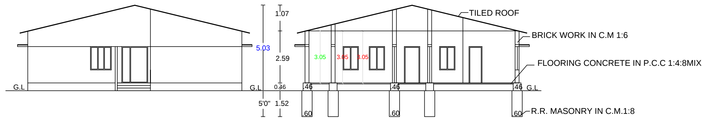
ELEVATION
