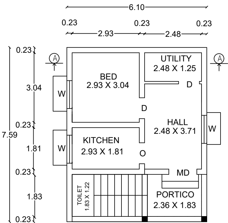
DR PLAN
