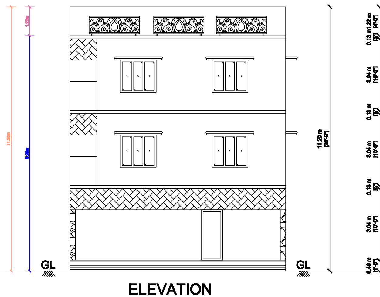
ELEVATION
