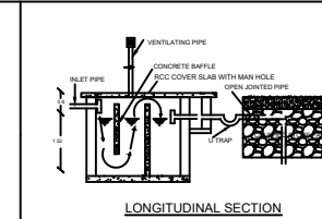
LONGITUDINAL SECTION
