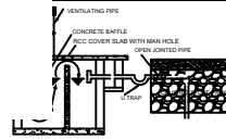
LONGITUDINAL SECTION
