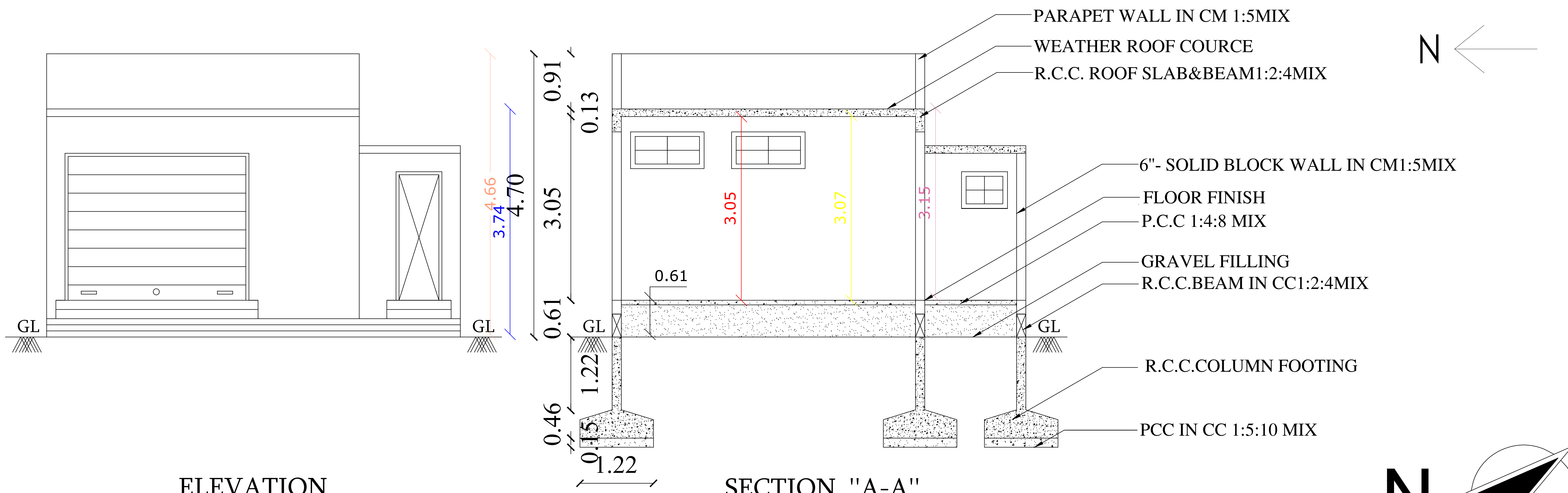
ELEVATION
