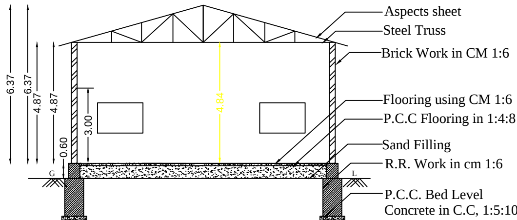
SECTION A-B
