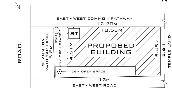
SITE PLAN SCALE : 1:100
