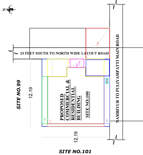
SITE PLAN SCALE 1:100
