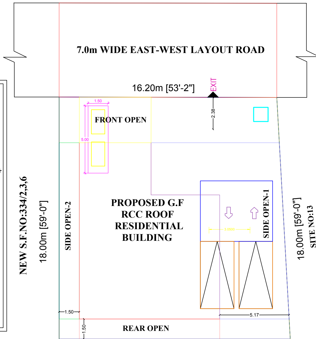
17.20m [56'-6"] SITE NO:10,11 SITE PLAN
