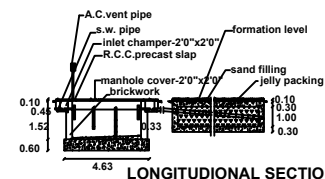
LONGITUDINAL SECTION
