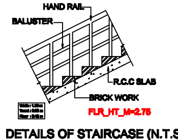
DETAILS OF STAIRCASE (N.T.S)
