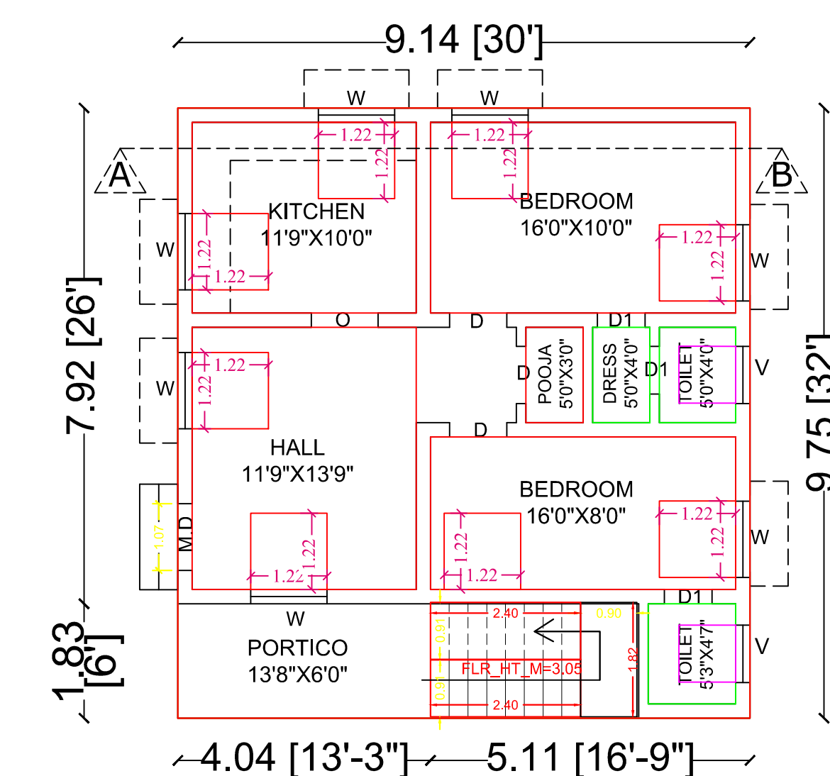
DOOR PLAN
