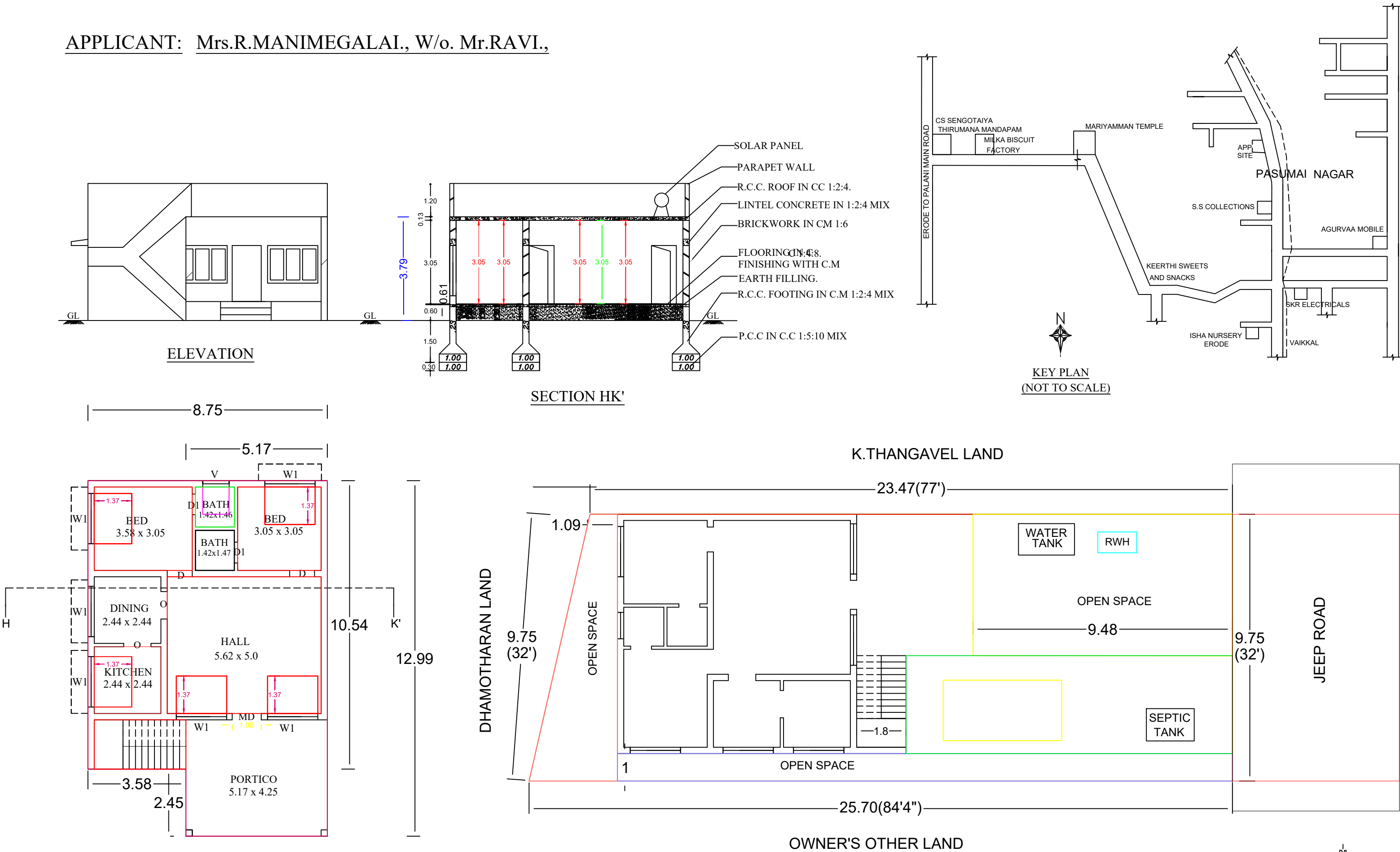
SITE PLAN SCALE 1:1
