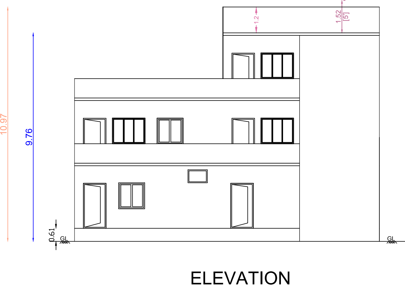
ELEVATION
