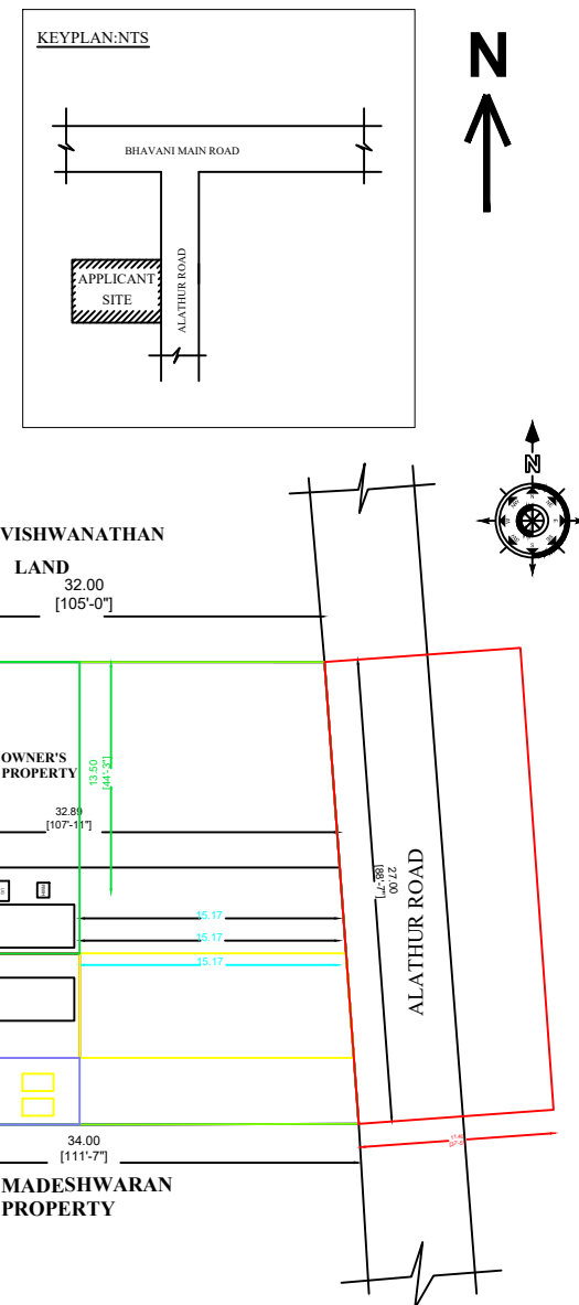
SITE PLAN ( Scale : 1:150)
