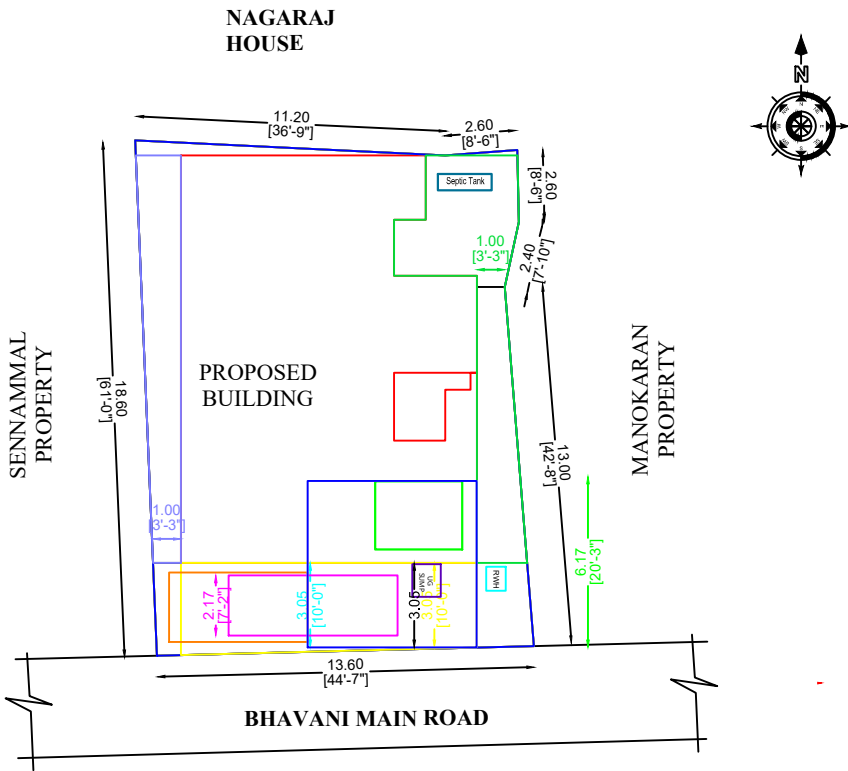
SITE PLAN ( Scale : 1:150)
