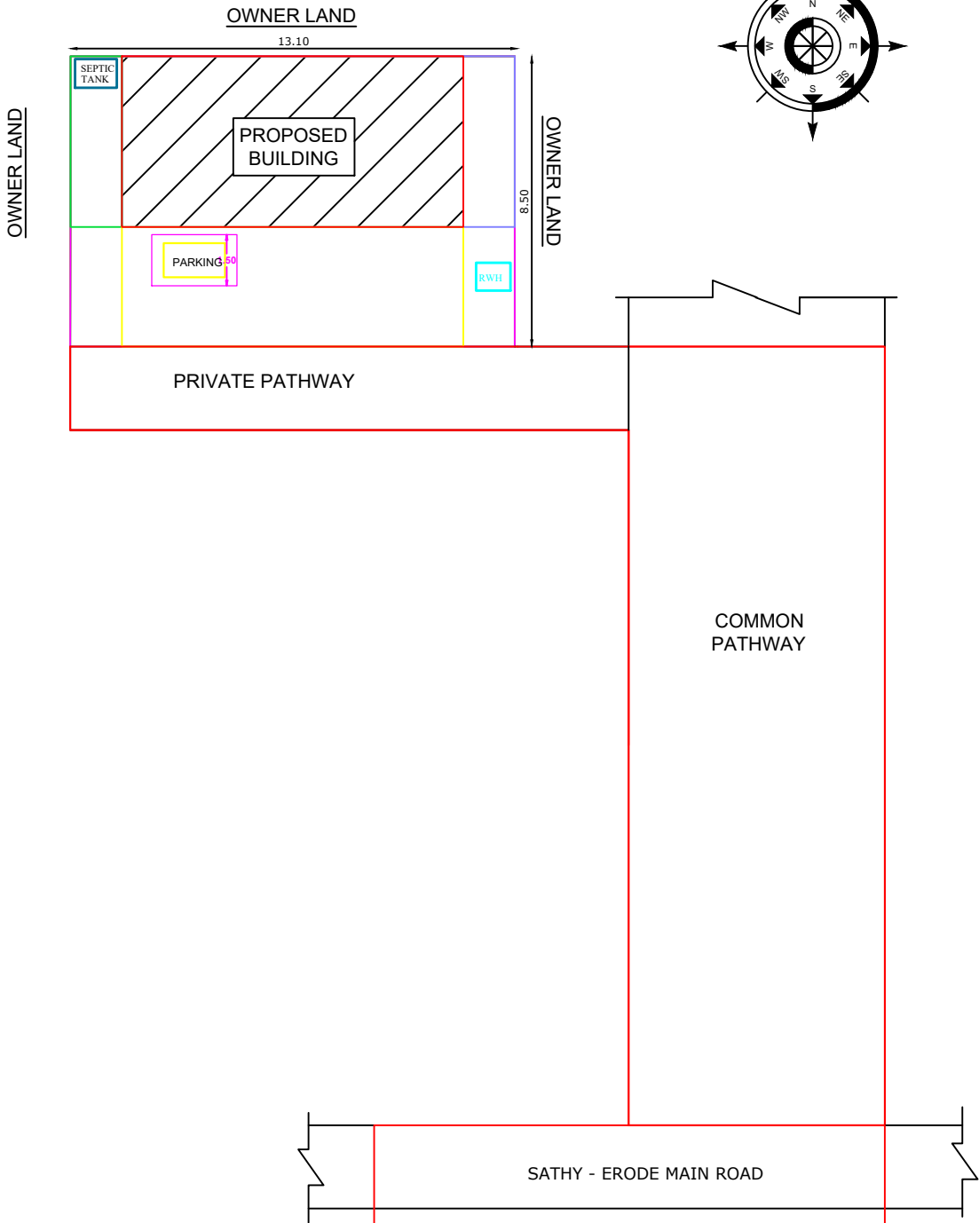
SITE PLAN (1:200)
