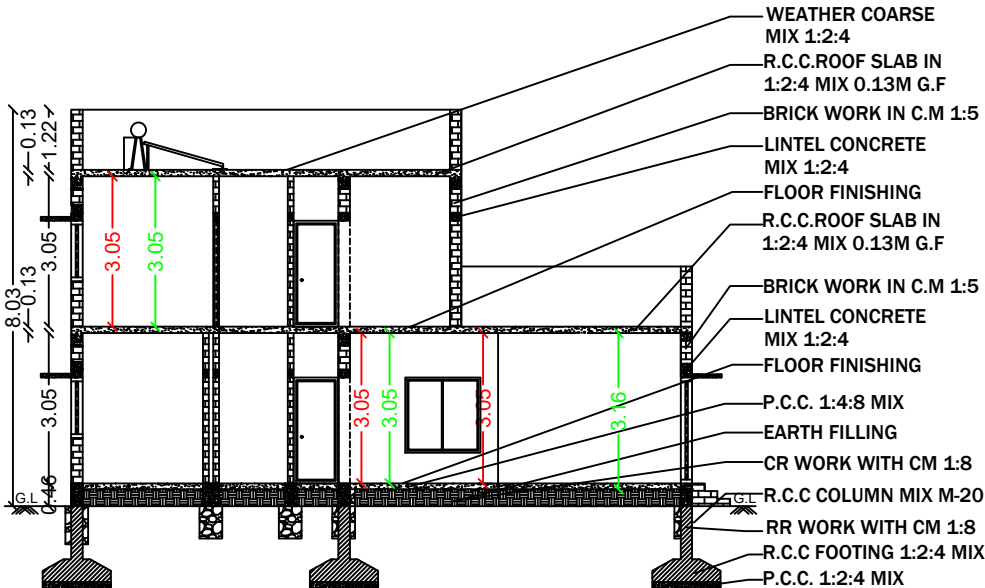
SECTION - AB
