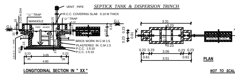
LONGITUDINAL SECTION IN " XX "
