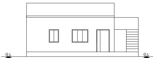
ELEVATION
