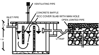
LONGITUDINAL SECTION
