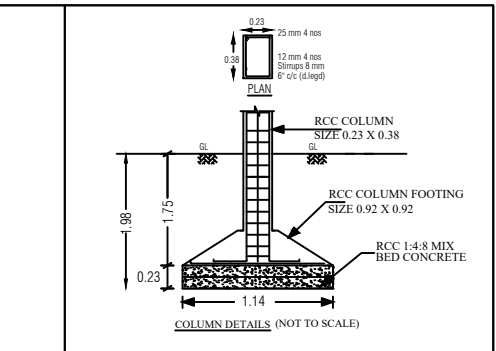
LONGITUDINAL SECTION
