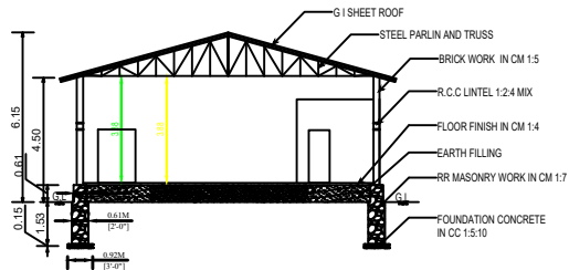
SECTION -LS
