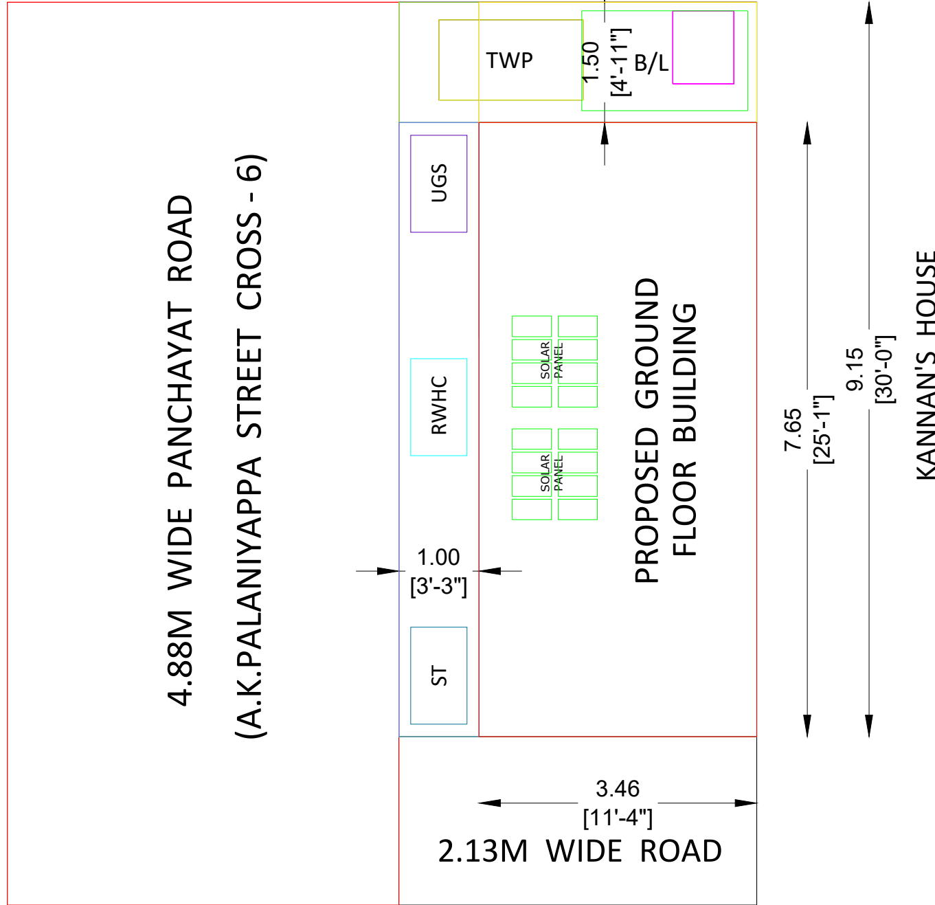
SITE PLAN 1 : 100
