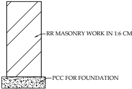
FONDATION DETAILS
