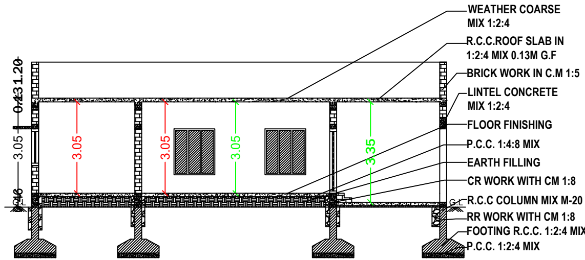
SECTION - AB
