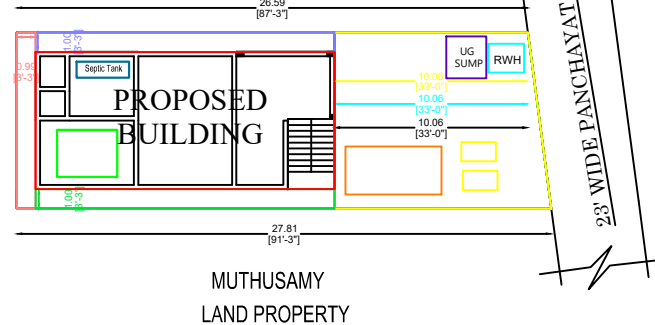
SITE PLAN ( Scale : 1:100)
