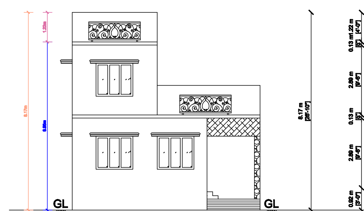
ELEVATION
