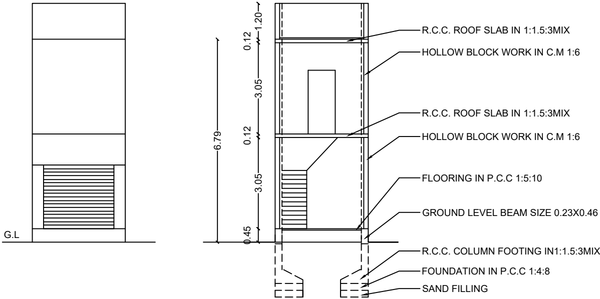
ELEVATION
