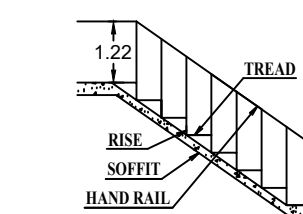
RISE : 17.5 CM TREAD : 25.0 CM WIDTH : 91.0 CM
