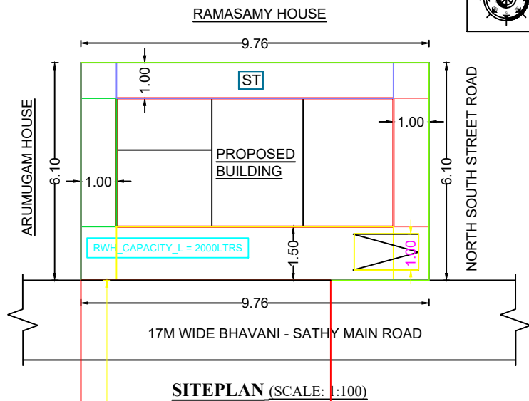
SITEPLAN (SCALE: 1:100)
