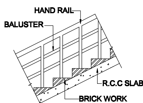
DETAILS OF STAIRCASE (N.T.S)
