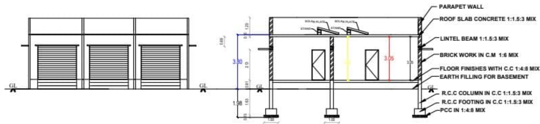
ELEVATION
