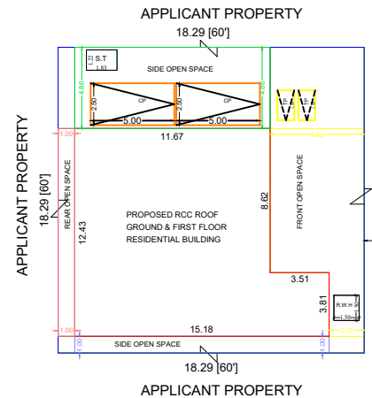
SITE PLAN SCALE- 1:150
