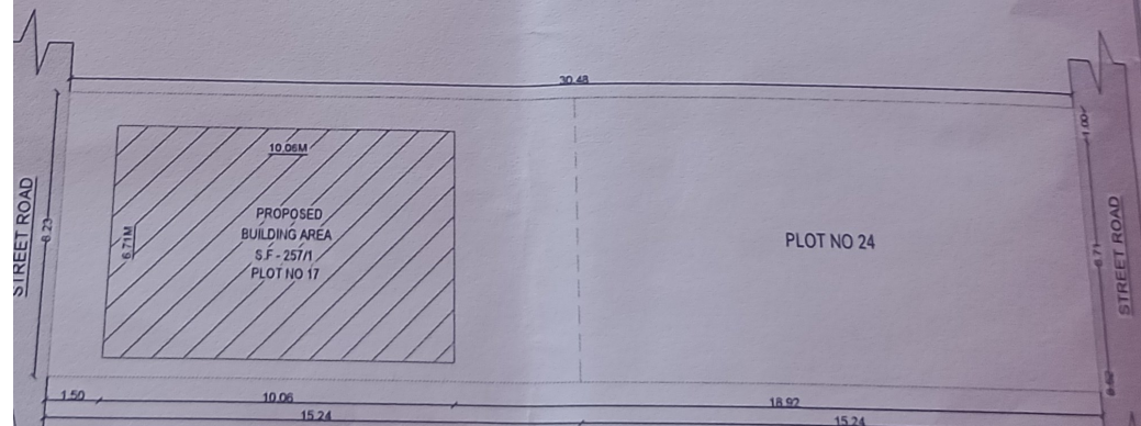
SITE PLAN SCALE 1:100
