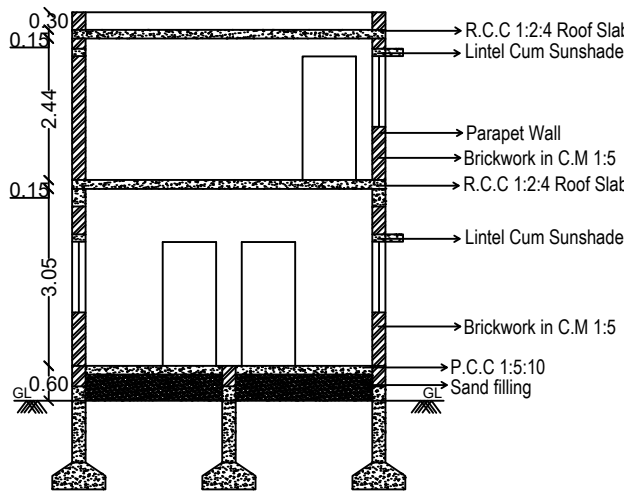
SECTION - AB
