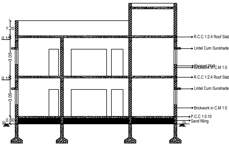
SECTION - AB
