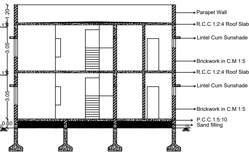
SECTION - AB
