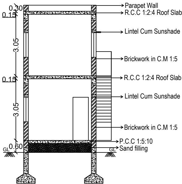
SECTION - AB
